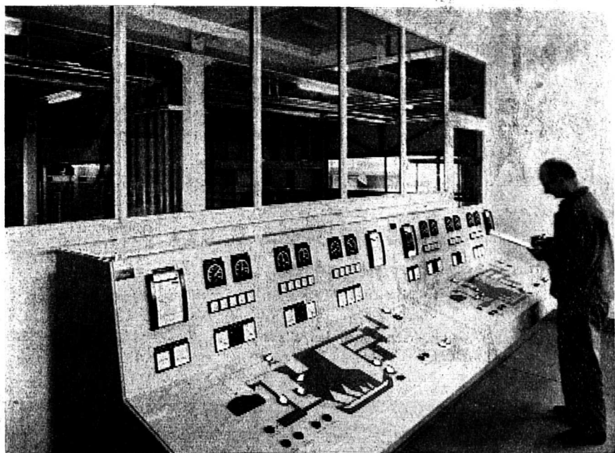
Le poste de commande est placé au centre de l'usine et permet l'observation simultanée des deux fours.
