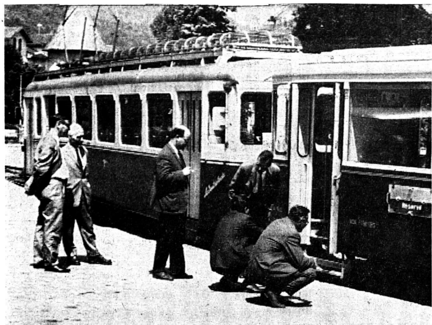
A l'arrivée à Monthey, quelques spécialistes examinent les bogies des nouvelles voitures, bogies dont la conception dans la suspension est révolutionnaire.
