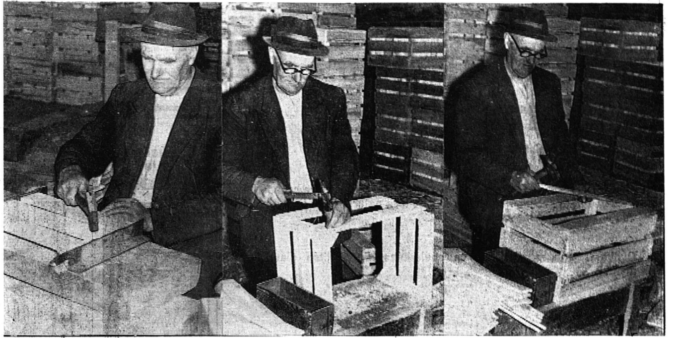
1. Sur un établi entre deux pièces d'acier, M. Udressy place les têtes, c'est-à-dire les côtés les plus étroits de la caisse. 2. Ensuite, la seconde pose consiste à monter les « à-côtés » pour donner à la caisse sa forme définitive. 3. La troisième et dernière phase de la fabrication c'est la pose du « fond ».
