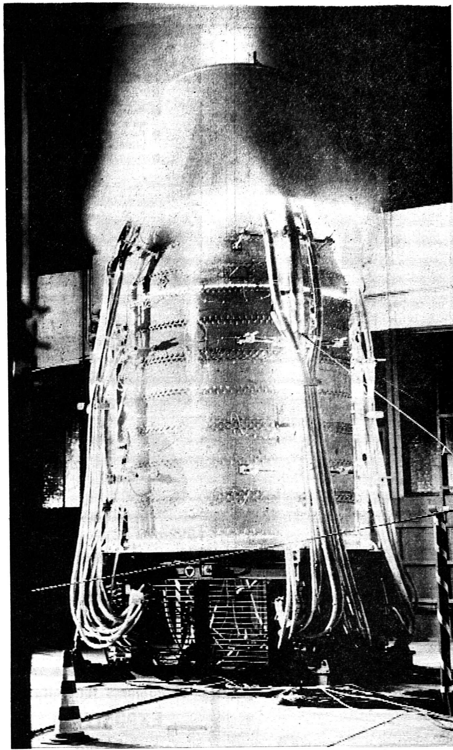
Essais de la coiffe protectrice du satellite qui sera lancé par la fusée Europa-1 (photo ELDO).
