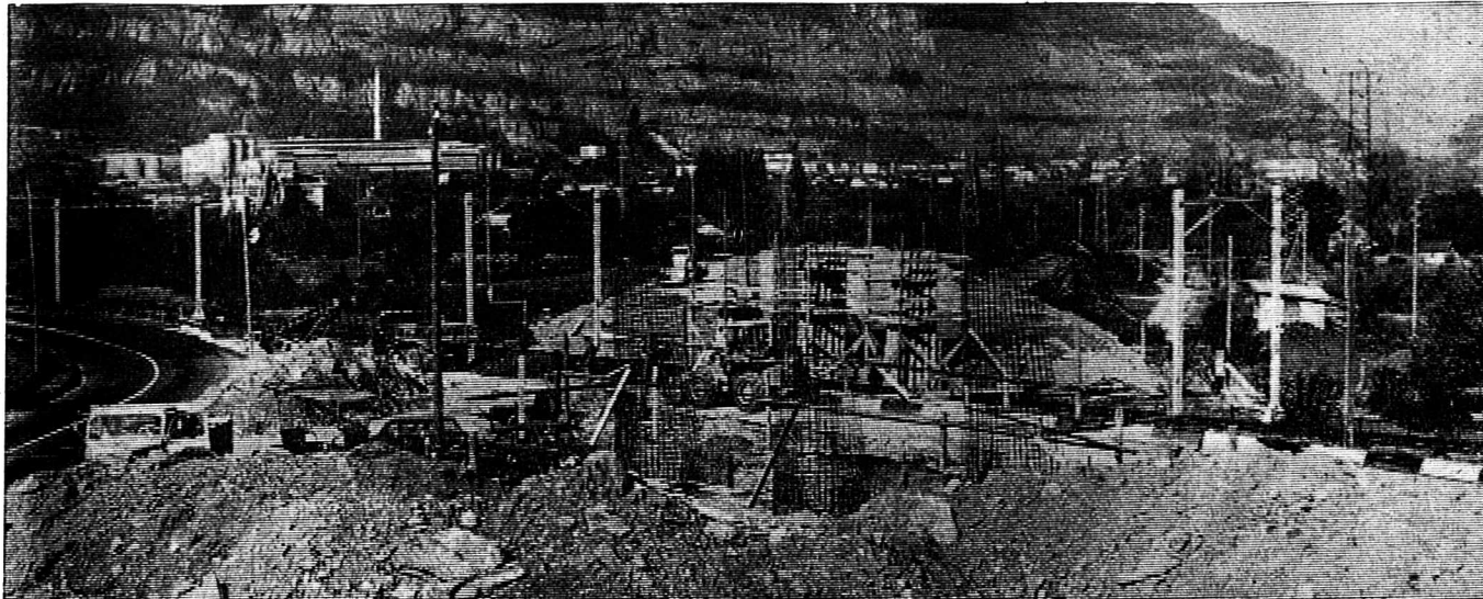
SAINT-MAURICE — Le nouveau tracé de la route cantonale Evionnaz-St-Maurice se dessine sérieusement au Bois-Noir. Ces jours, l'entreprise de maçonnerie a mis en chantier le ferrailage et le coffrage des piliers qui supporteront le tablier du pont en enjambant la voie de chemin de fer tandis que, de chaque côté, on continue à amener des matériaux qui sont tassés aux vibreurs. Si le temps reste au beau, nul doute qu'à la fin de cette année une bonne partie du gros œuvre de cet ouvrage sera terminé. NOTRE PHOTO : une vue du chantier en direction de Saint-Maurice.
