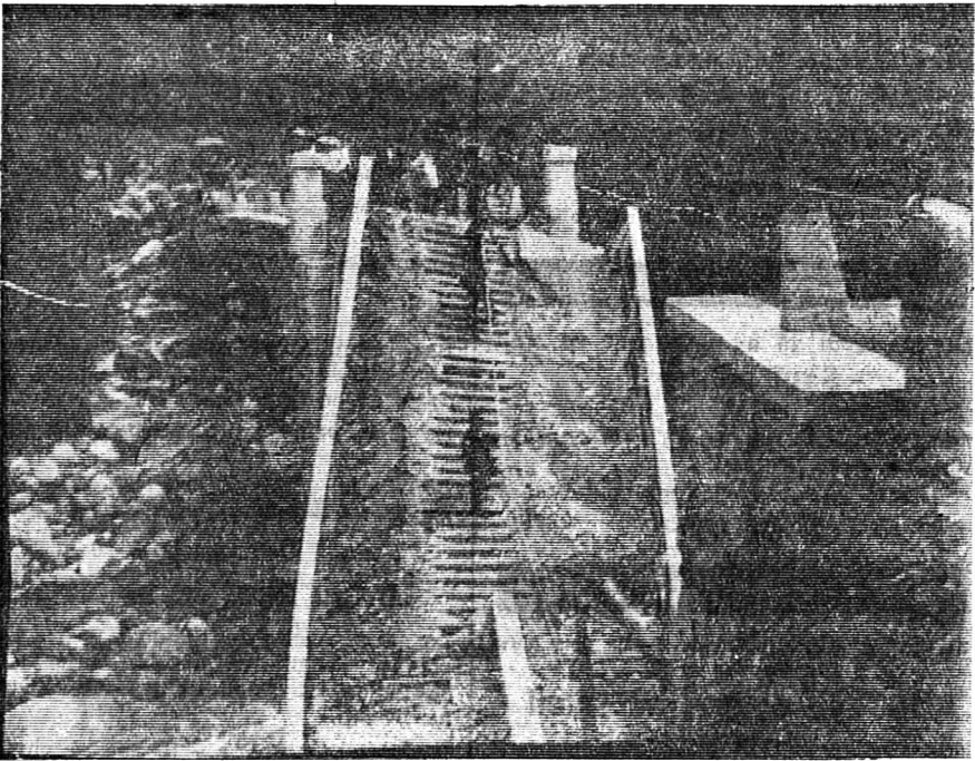
Le 7 juillet 1902, la culée aval du pont sur le Durnant n'a pas résisté: le tablier s'est effondré dans le lit du torrent. On avait alors placé des escaliers en bois pour permettre aux piétons de circuler.
