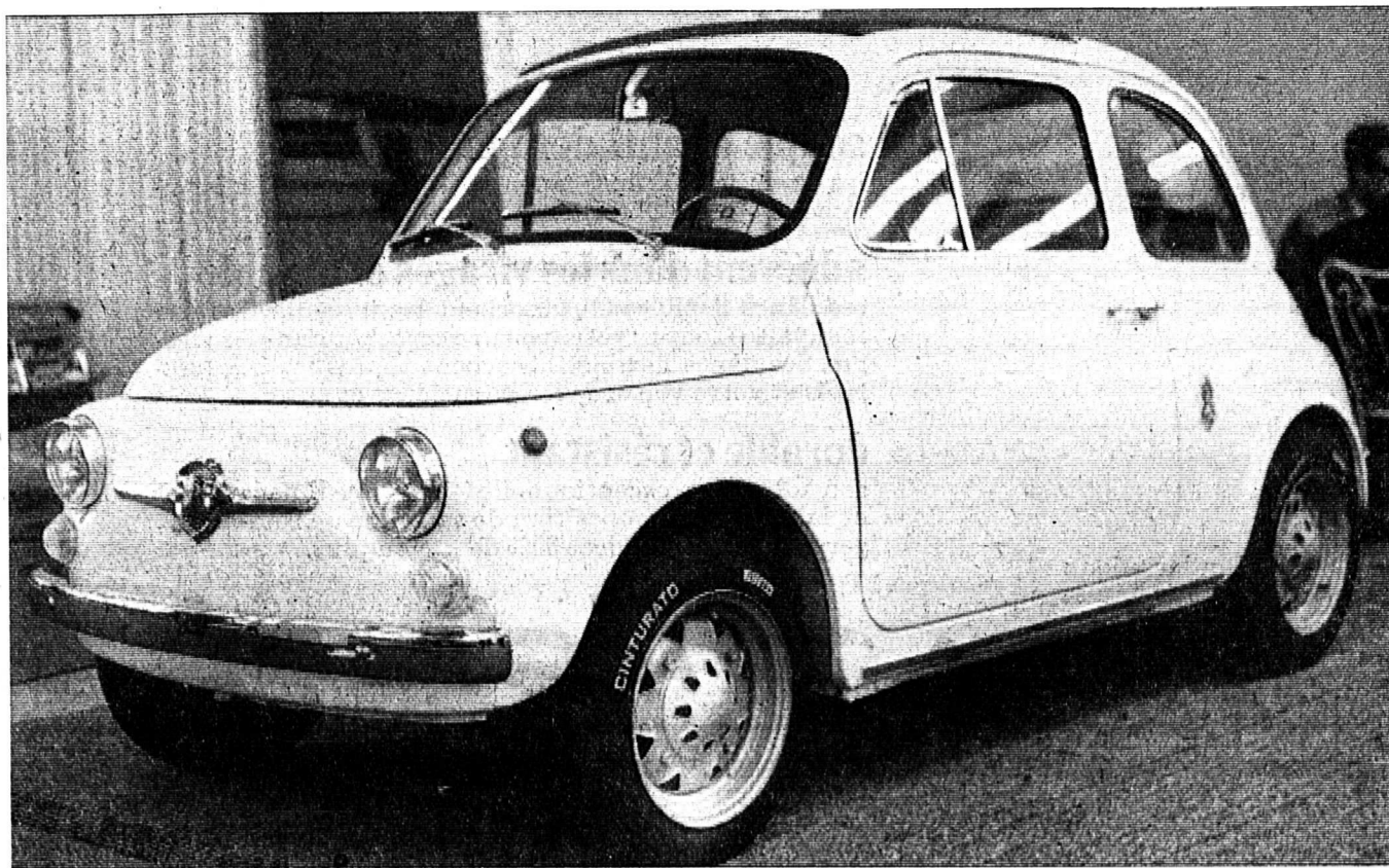
FIAT-ABARTH 695 SS — Variante sportive de la Fiat Abarth 695. Mêmes caractéristiques que Fiat-Abarth 695, sauf : moteur 38 ch. (DIN) à 5200 tr/mn; 55,2 ch/L (DIN); exig. en oct. supercarburant. 1 carburateur inversé Solex PBIC 34. Vitesse max. 140 km/h (usine).
