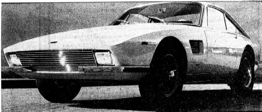
LA T.V.R. TRIDENT a été dessinée par « Fiore » (Paris) et exécutée par la carrosserie Fissore. Pourvue d'un moteur Ford V-8 de 4,7 l. développant une puissance de 270 CV au frein à 7000 tours/min., elle peut atteindre la vitesse de 240 km/h. Elle est pourvue d'une boîte Borg-Warner à quatre vitesses, toutes synchronisées, et bientôt, sur demande, d'une boîte automatique. Elle est exposée au stand du carrossier Fissore.
