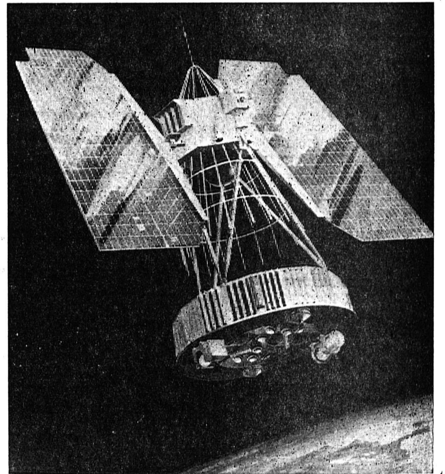
Le satellite météorologique « Nimbus A »
