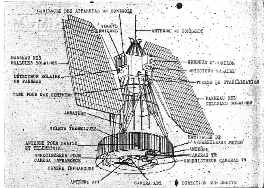
Schéma de « Nimbus A »
