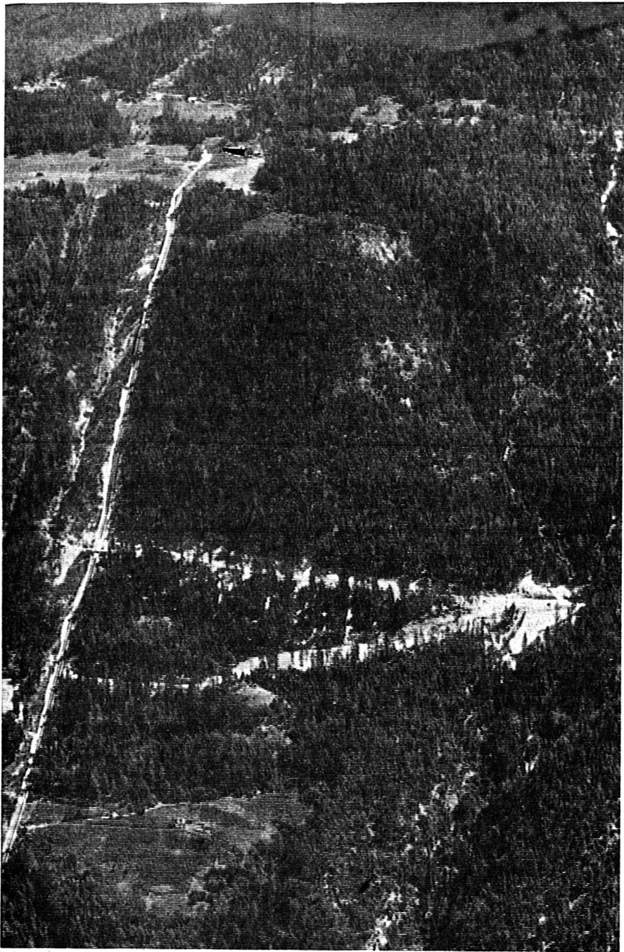
La route des Mayens de Riddes progresse lentement mais sûrement. Lacets et tunnels se succèdent déjà. Actuellement, l'on achève le gros œuvre d'un nouveau franchissement de la double conduite forcée de l'usine d'Ecône. Au sommet de cette photo aérienne, ce sont les mayens...
