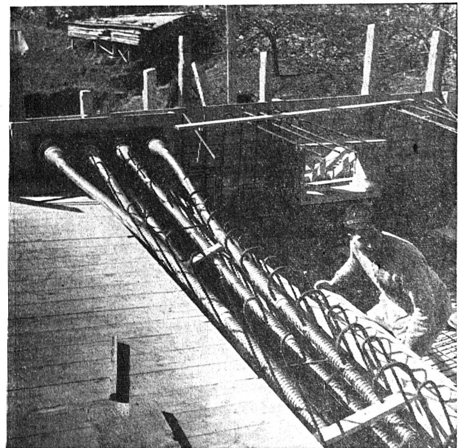
Au cours des travaux, on assiste ici au ferrailage et à la mise en place de câbles de la précontrainte.
