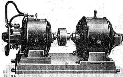
Moteurs à courant alternatif accouplés directement avec une dynamo à courant continu à basse tension.
