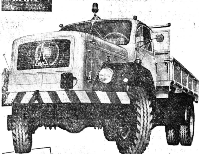
Modèle JUPITER 195-AK à moteur Diesel 8 cylindres, de 195 CV-DIN, refroidissement à l'air, poids total 16 tonnes. Largeur pour la Suisse 2300 mm
