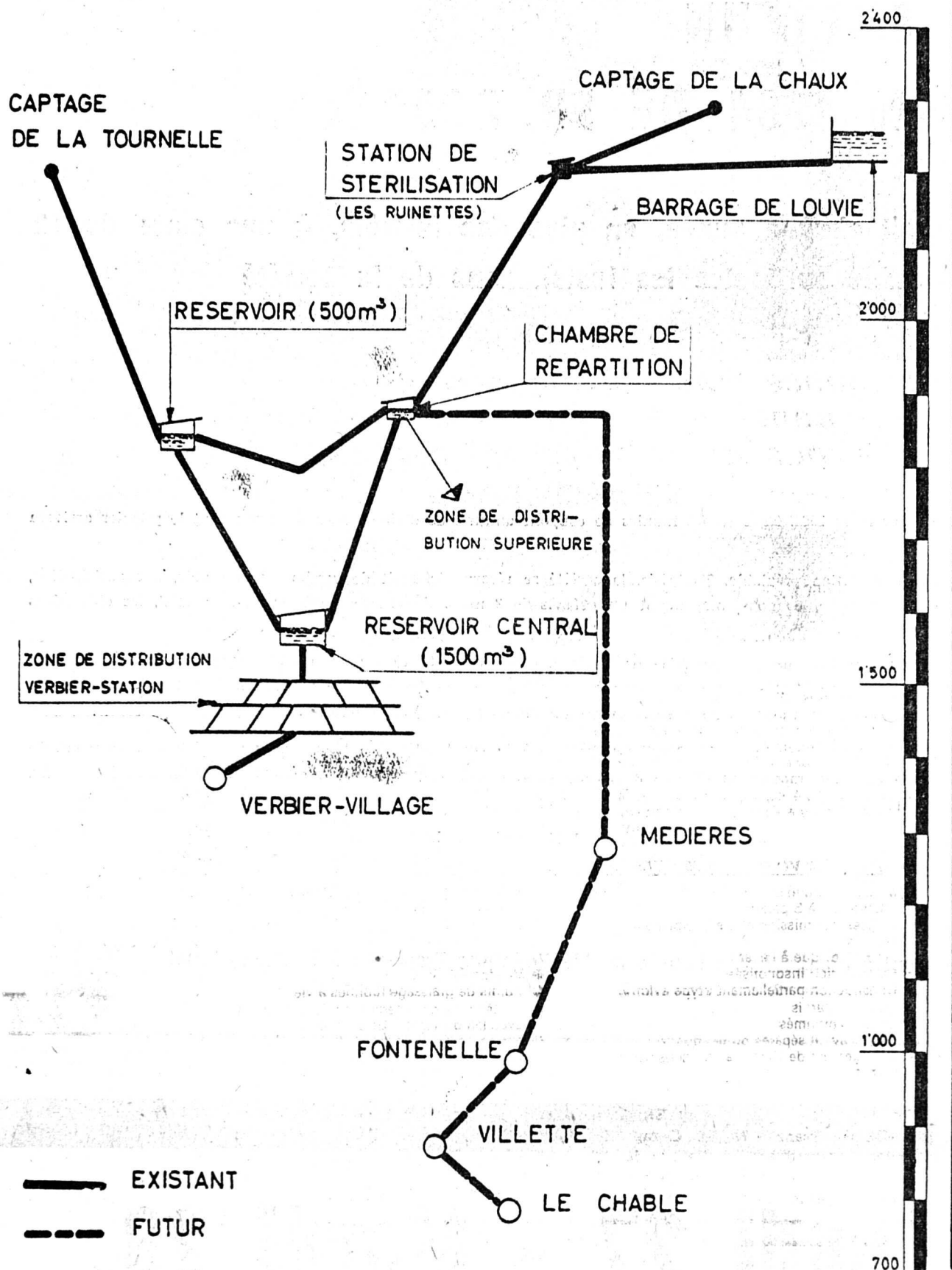
Plan de situation du réseau d'eau potable de la région de Verbier.
