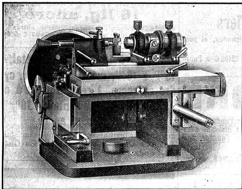
Machine à pivoter semi-automatique
