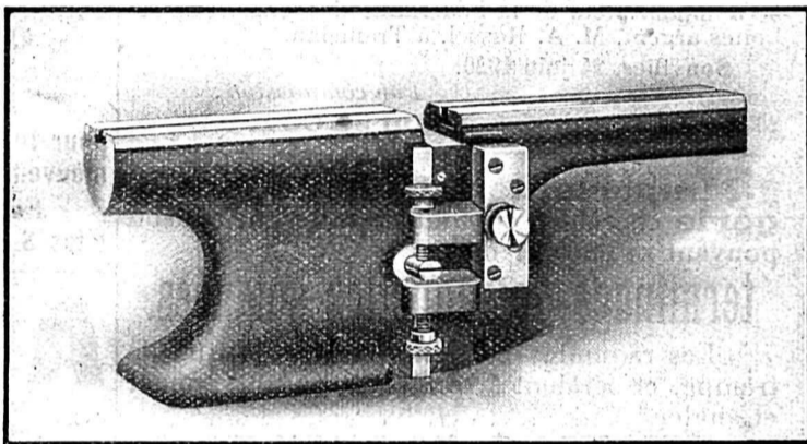
Banc mobile, pour le centrage rigoureux des forets, pointes, etc.
