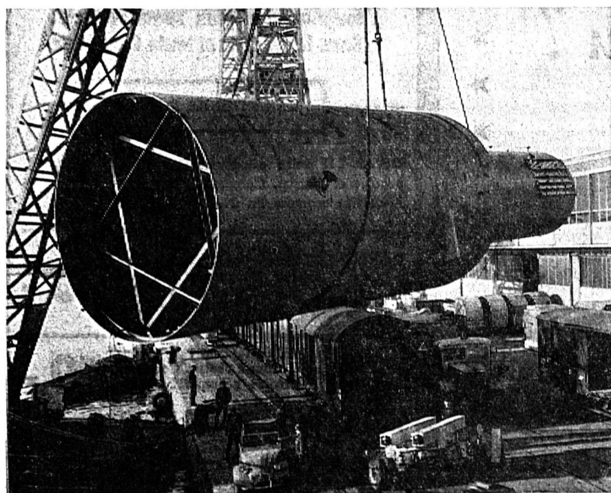
C'est dans le port de Marseille, ainsi que nous l'avons déjà annoncé, que le bateau français « Gyptis » a déchargé les éléments principaux du « manteau » de la tour de distillation atmosphérique de la raffinerie de pétrole de Collobey. Ces pièces lourdes et volumineuses sont conduites en Suisse par trains routiers. Voici une phase de ce débarquement délicat. (Photo S.I.R.R.)
