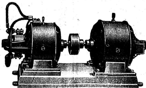
Moteur à courant alternatif accouplé directement avec une dynamo à courant continu à basse tension.
