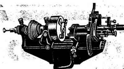
Machine à replanter
