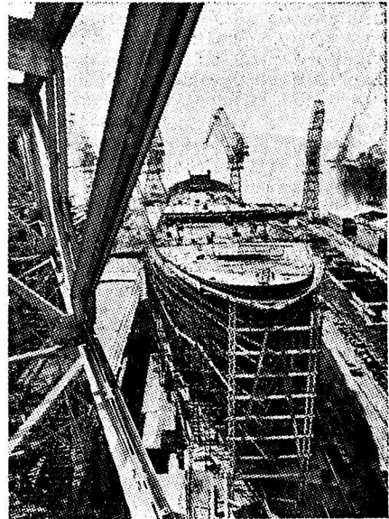
Le navire étend toute la longueur de ses 210 mètres sur la cale sèche. Les échafaudages entourent encore la coque. Ils ne disparaîtront qu'à la veille du lancement, une fois donné le dernier coup de pinceau
