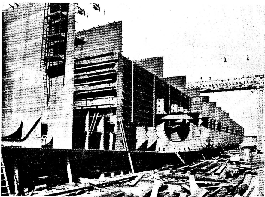
Des cloisons transversales divisent le pétrolier en une série d'alvéoles latérales, qui assurent la rigidité de la coque. Au centre, les évidements nécessaires sont réservés pour les machines et les réservoirs à pétrole
