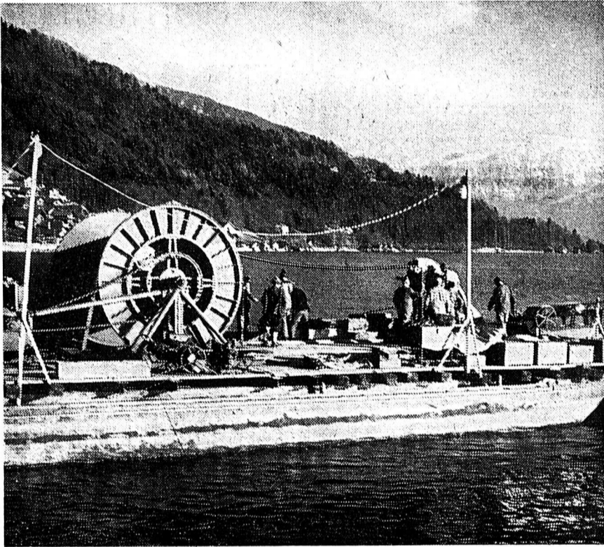
Un câble pour l'électricité a été immergé par un bateau dans le lac de Thoune
