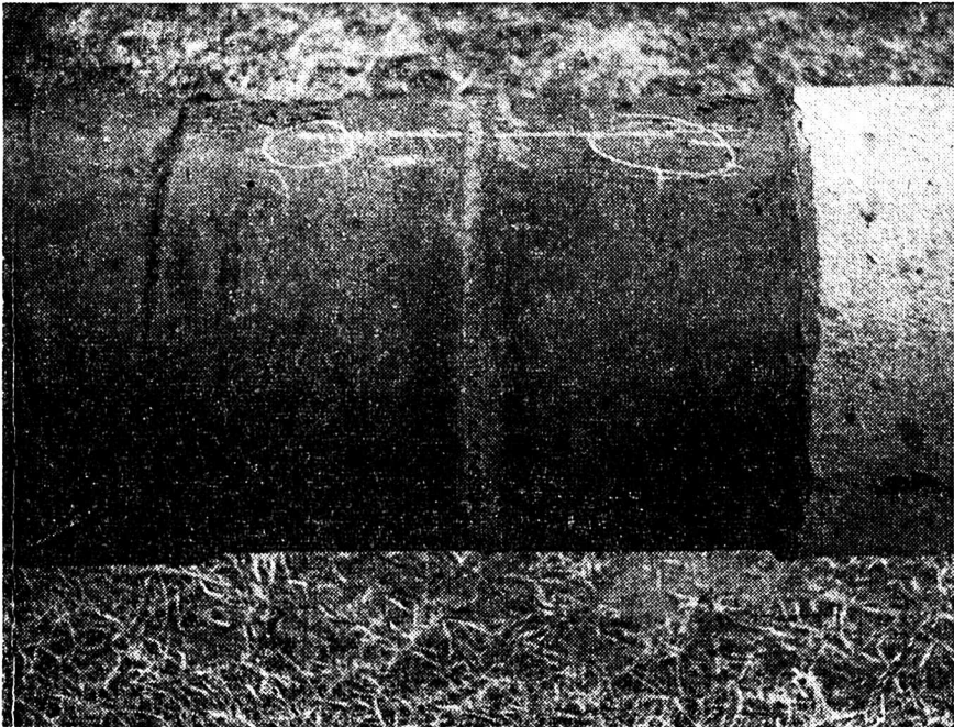
Un détail de la soudure entre deux tuyaux.
