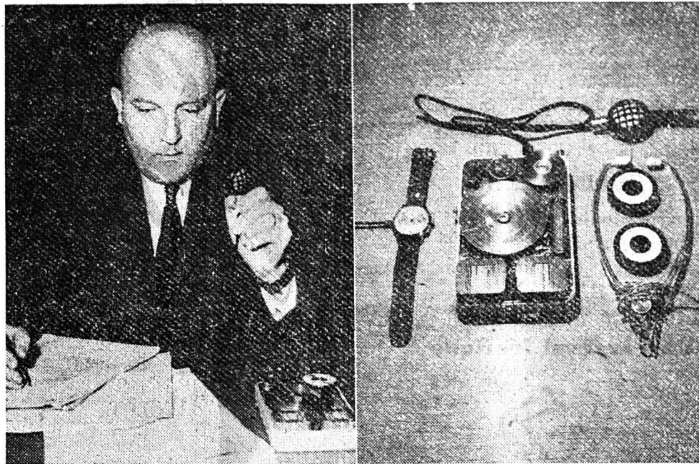
Le « Miniphone » est un appareil enregistreur sur fil d'acier de format très réduit. Notre photo montre à gauche l'appareil fonctionnant aussi bien avec une pile qu'avec le courant ordinaire. A gauche le microphone montre-bracelet, au milieu l'appareil de réception avec microphone de main (en haut) à droite l'écouteur avec deux bobines de fil d'acier, chacune pour un enregistrement d'une heure.
