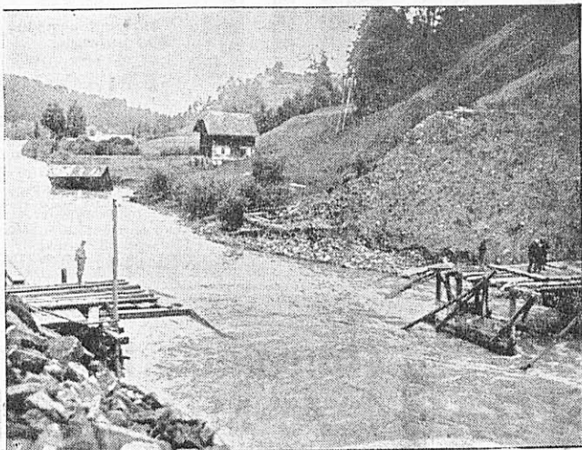
Une vue du pont de service de Corbières emporté il y a quelques jours par une crue subite de la Sarine. Actuellement, les travaux de remise en état sont très avancés.
