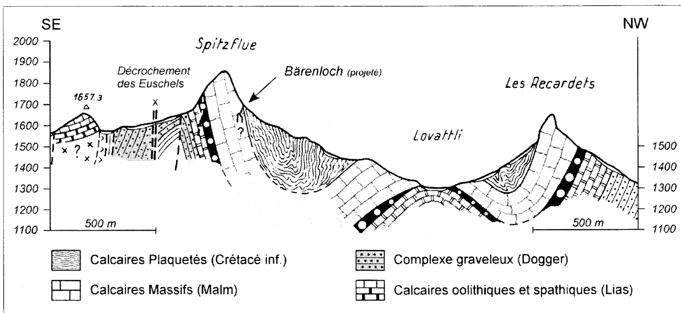
Figure 1 : Coupe géologique de la région de la Spitzflue (modifié d'après ANDREY 1974)
