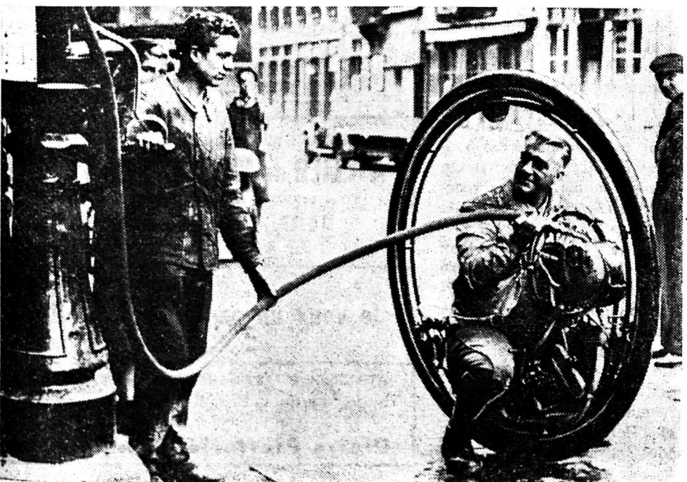
MUNICH La roue à moteur a séduit déjà plus d'un inventeur. Un Suisse, M. Gerber, installé dans la capitale bavaroise, vient de mettre au point cette machine qui peut atteindre une vitesse de pointe de 190 km.-h.
