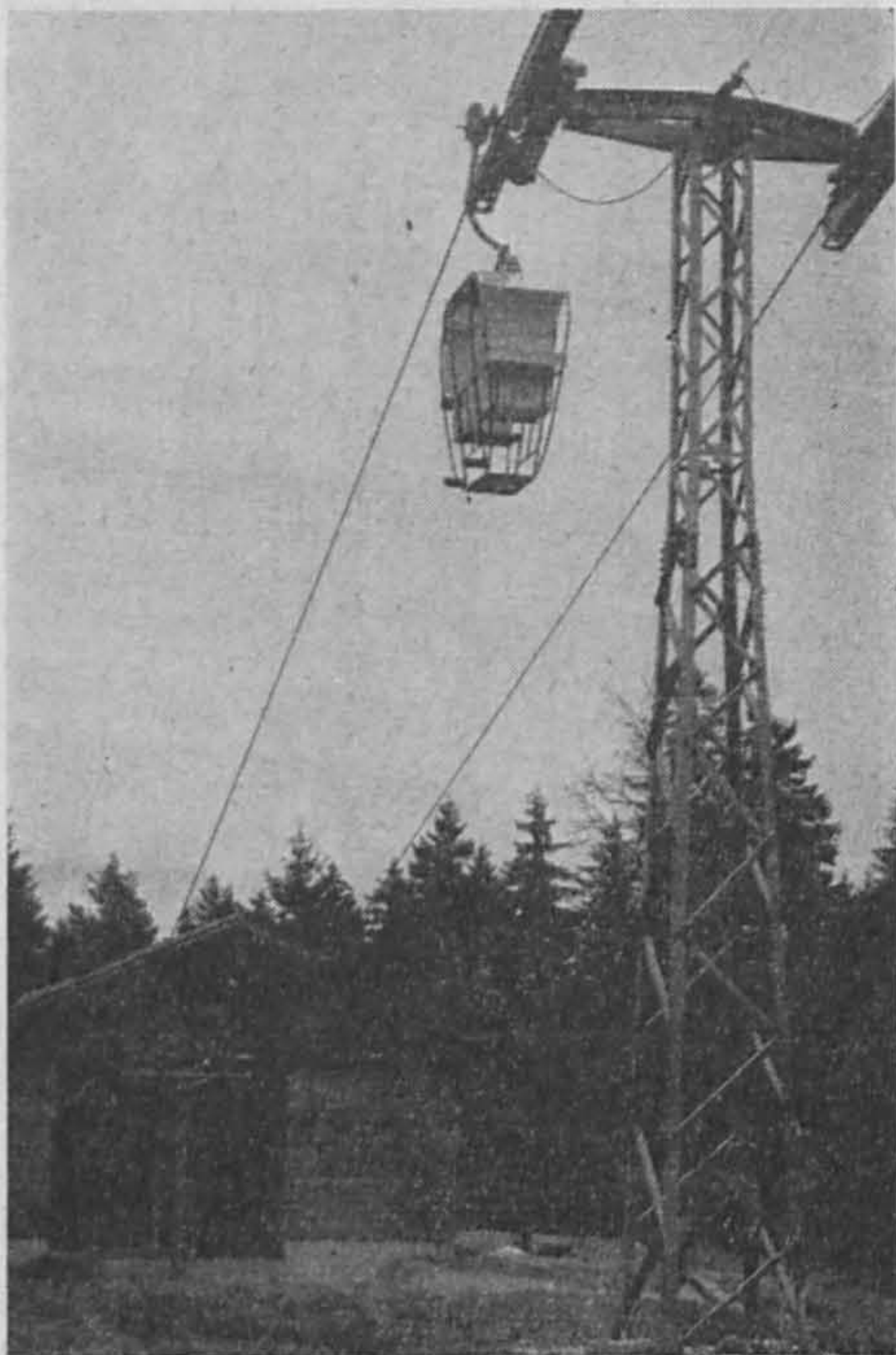
Le télécabine qui relie les Hauts-Geneveys à Tête-de-Ran.
