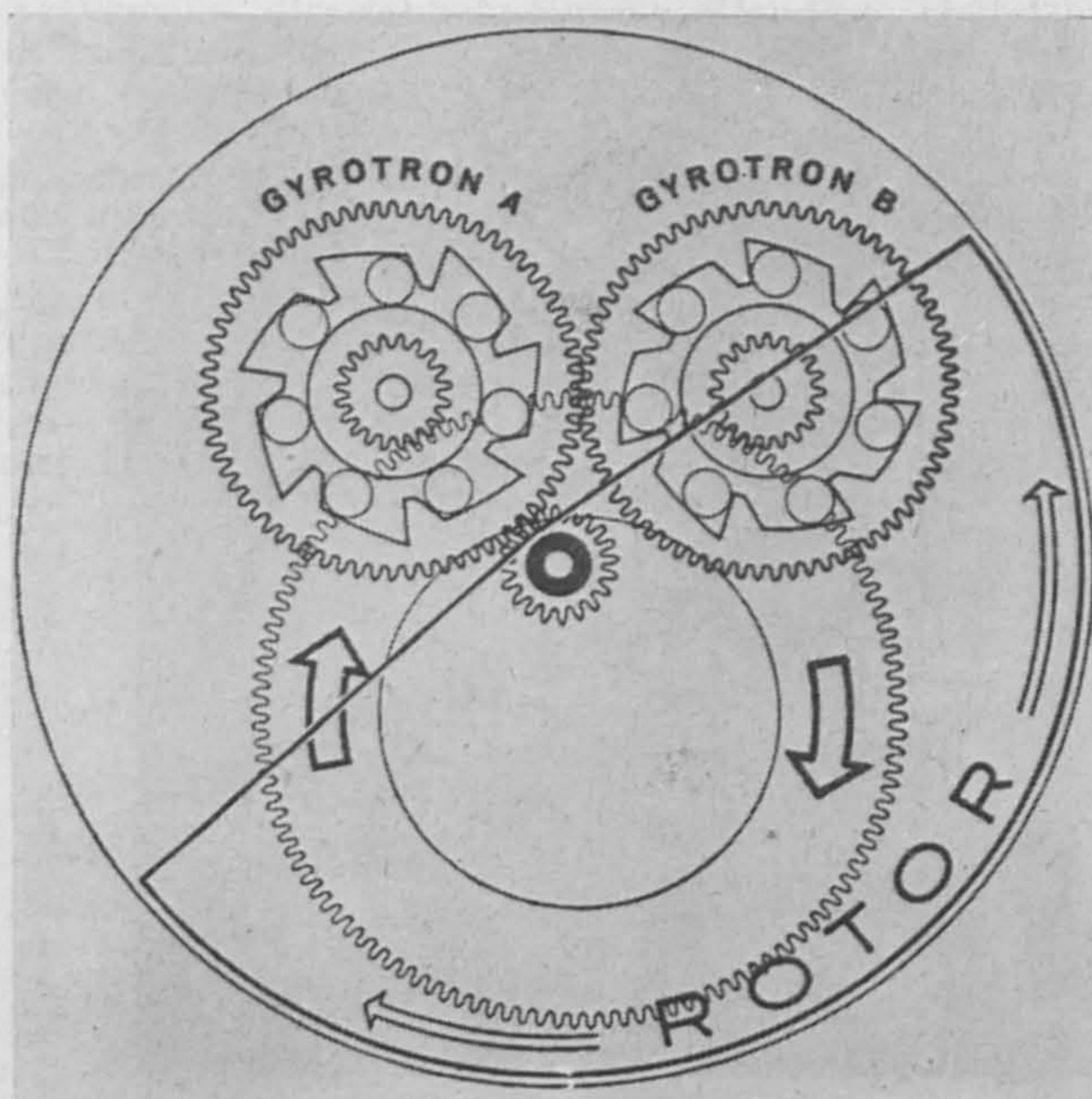
Dispositif de remontage automatique de la « gyromatic » de M. Pierre Graef.
