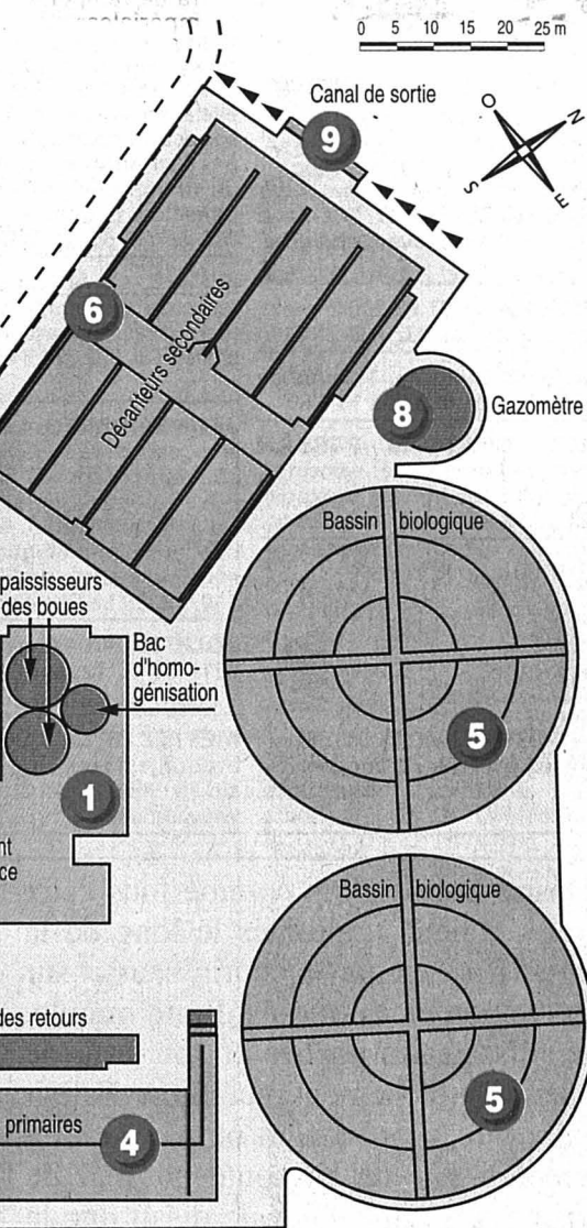
6 Décanteurs secondaires
