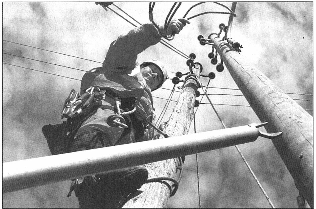
Dialogue du jeune et du vieux poteau.
