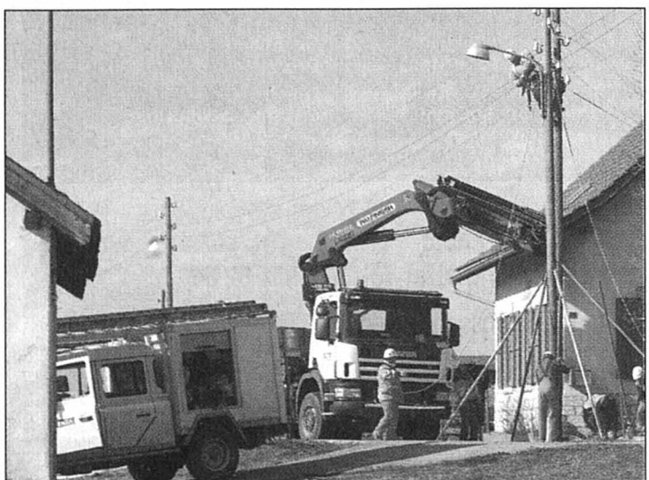
Le poteau, chose rare, alimente directement la maison par voie aérienne. Il supporte aussi un candélabre.
