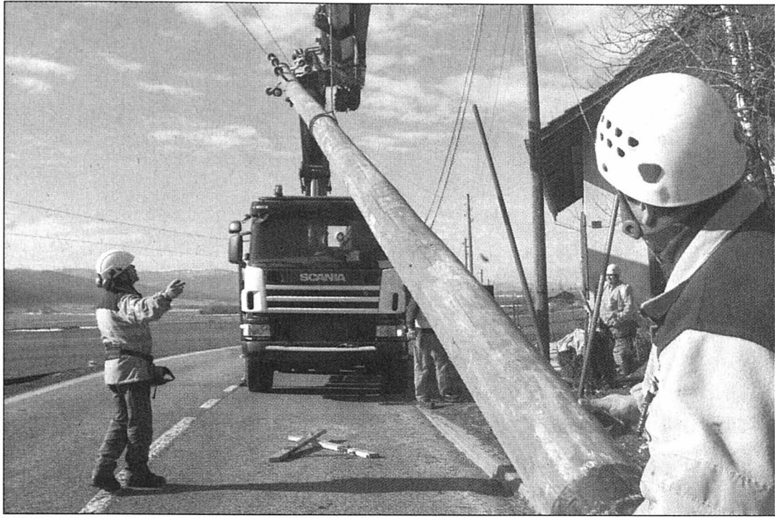
Déchargement du poteau neuf.
