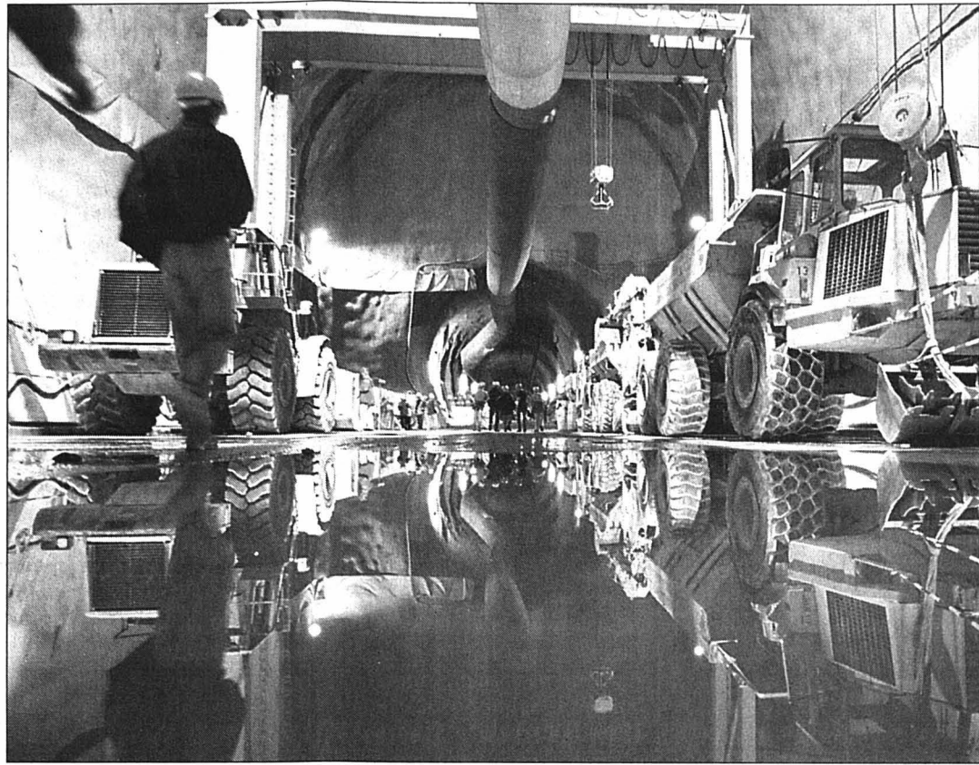
Le tunnel du Gothard devrait être mis en service en 2014. Ici, l'avancement des travaux au 30 août dernier.
