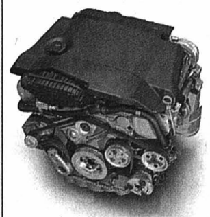
Le bloc-moteur V6 en fonte graphitée et compacte (CGI) est, avec 202 kg, le plus léger de ce type.
