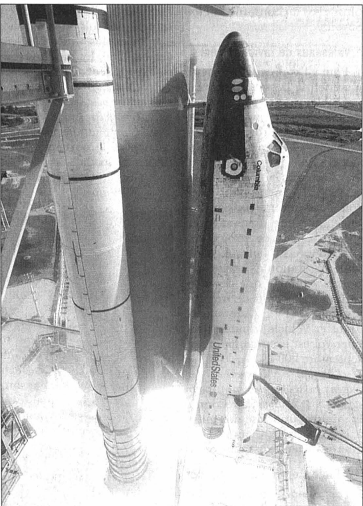
La navette Columbia photographiée lors de son départ le 16 janvier à Cap Canaveral. PHOTO KEYSTONE
