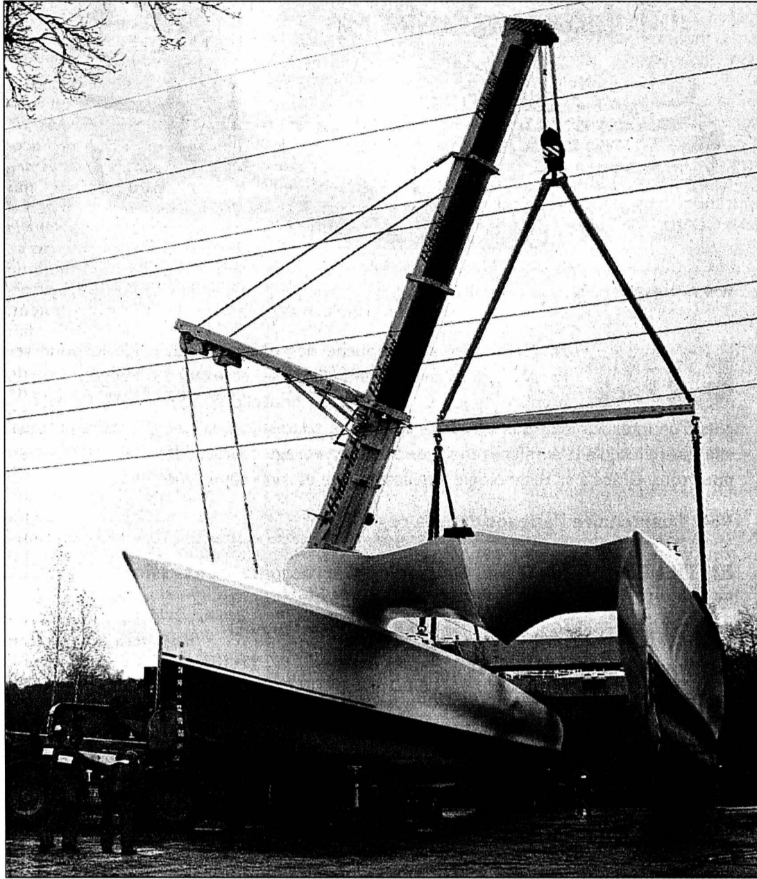
Une énorme grue a hissé, hier, les deux flotteurs de 46m de ce qui était l'Iris «New York» d'Expo.02.
