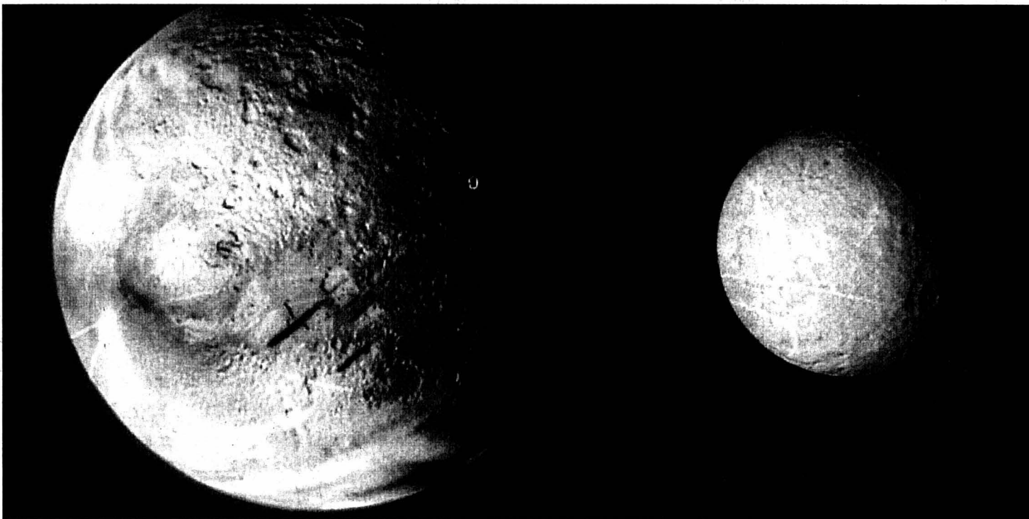
Ces portraits de Pluton et Chiron ne sont qu'une vue d'artiste. Même le télescope spatial Hubble ne distingue pas des détails inférieurs à 500 km!
