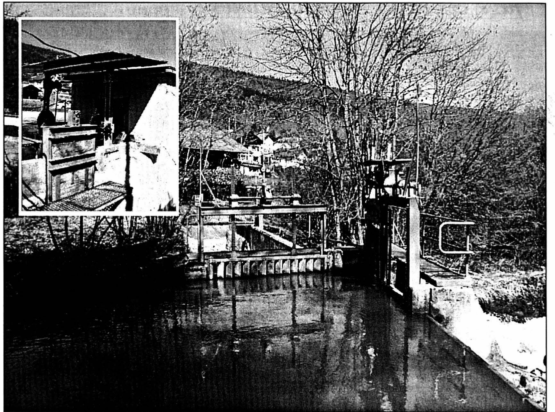
Sur la Suze, le départ du canal menant à la petite usine avec, en médaillon, le bâtiment abritant les installations techniques. PHOTO EGGELER
