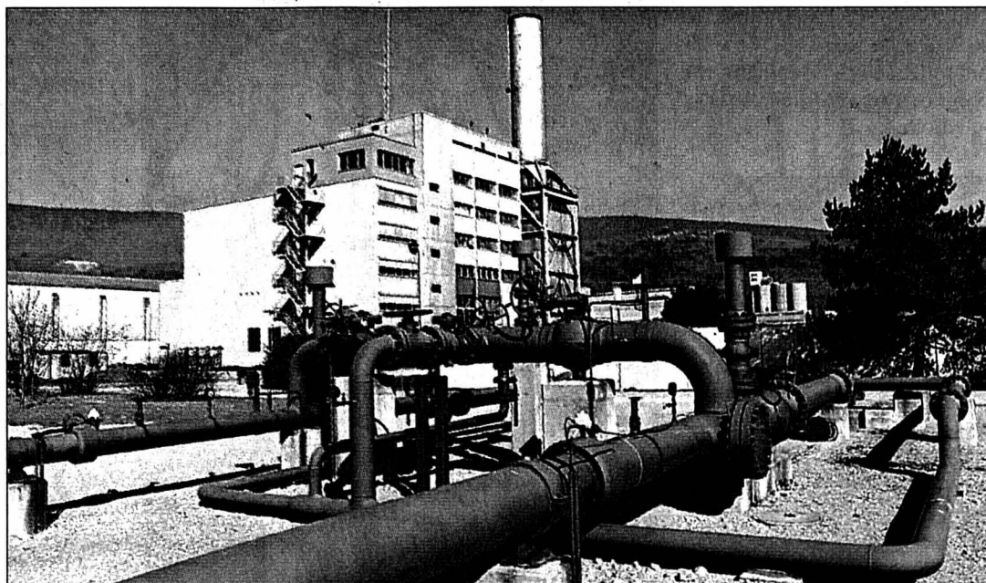
La station cantonale d'alimentation en gaz naturel de Cornaux avec, derrière, la centrale thermique.
