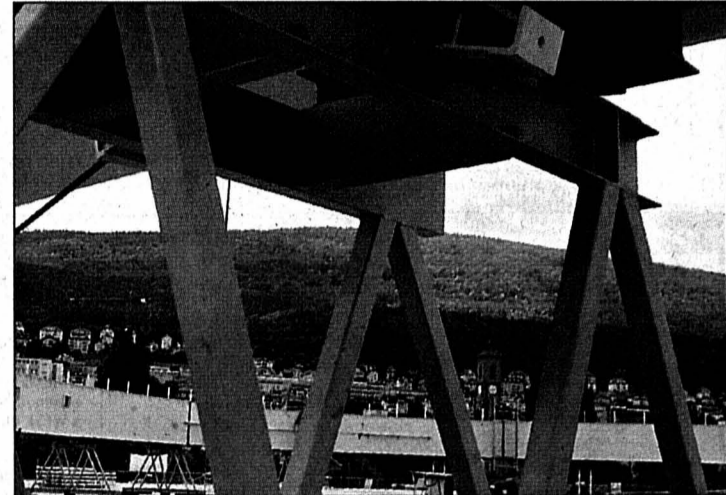
Vue partielle de l'un des chevalets métalliques qui font le lien entre la tête des pieux soutenant les galets (pieux qui ne sont pas les mêmes que ceux de la plate-forme) et les trois anneaux périphériques.
