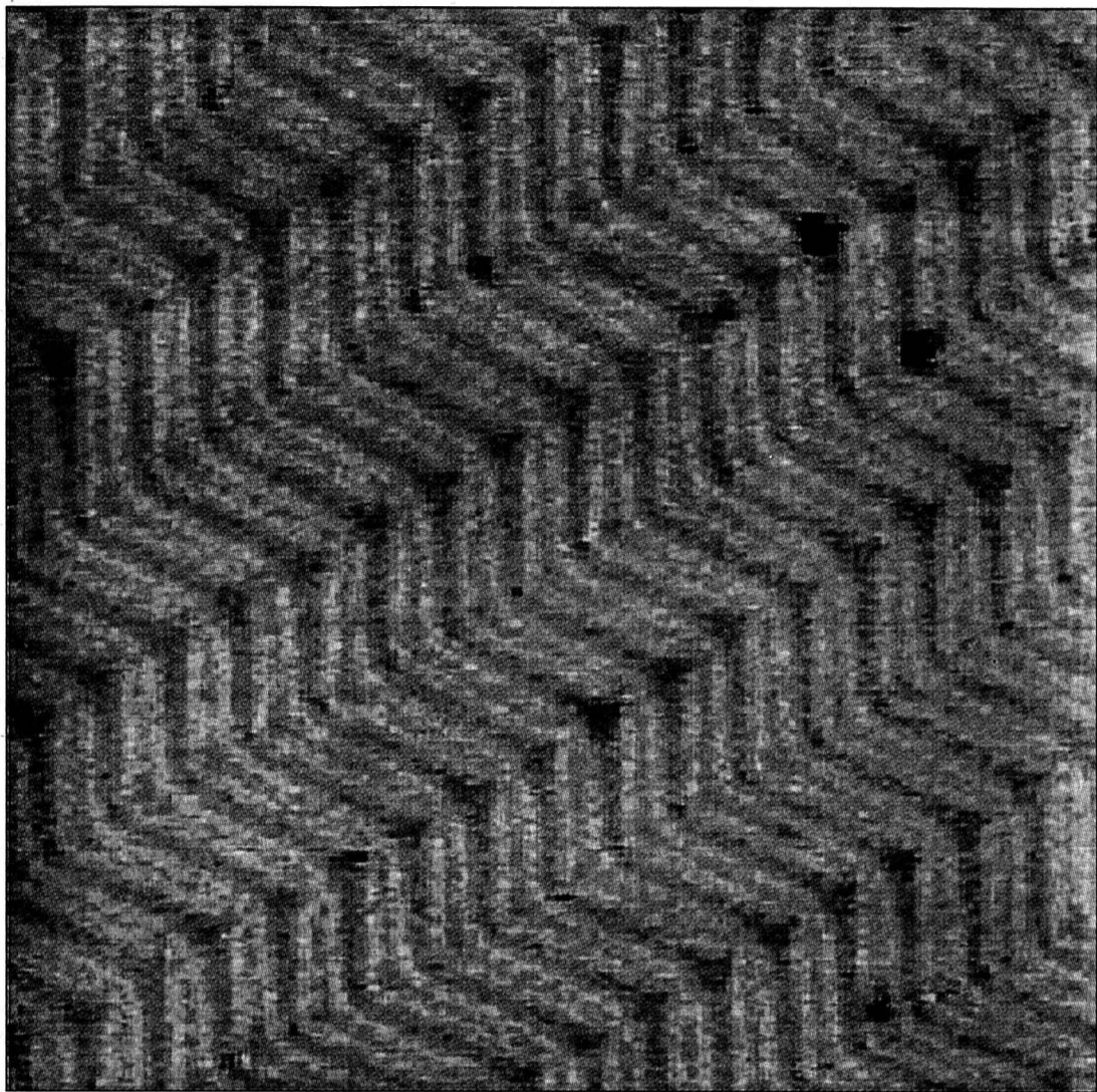
Le microscope à effet tunnel permet de visualiser la surface d'un cristal reconstruit en zigzag. Ces zigzags contiennent des défauts réguliers qui permettent « d'accrocher » des plots de Cobalt sur cette surface d'or. Chaque plot contient environ 200 atomes.
