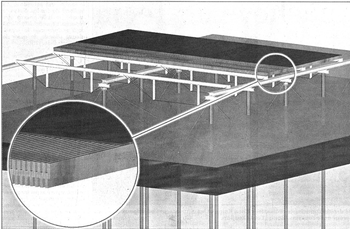
Une structure métallique sur pieux, soutenant un platelage de simples planches.
