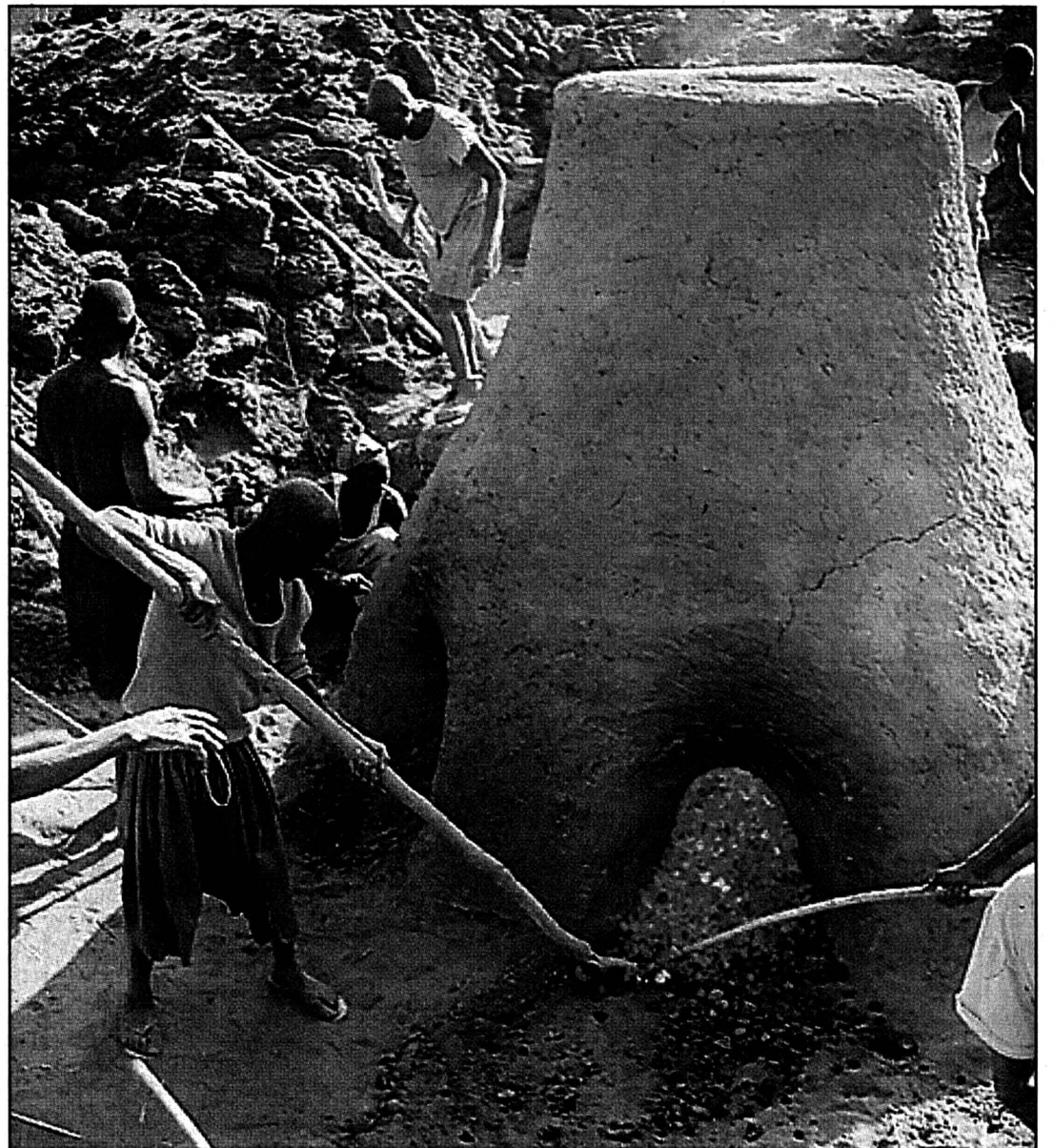
Four du Mali, la porte est dégagée et les scories coulent. L'éponge de fer qui résulte de cette extraction sera encore martelée pour livrer son précieux métal photo Eric Huysecom
