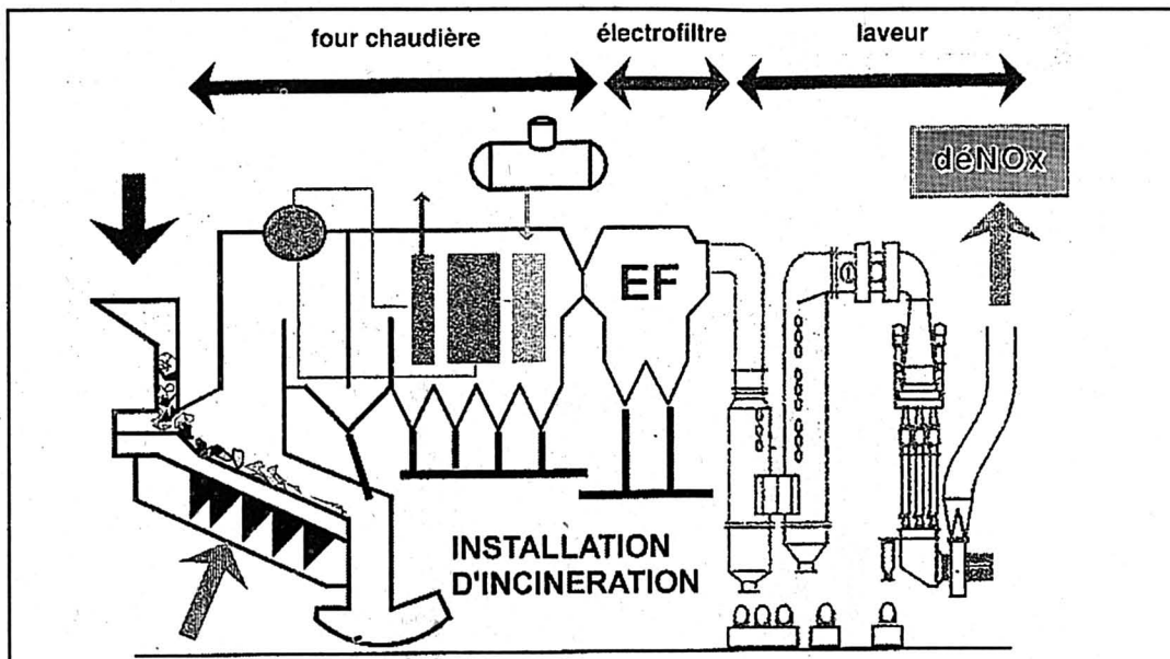
Avec le système choisi, la dénitrification sera placée en fin de circuit du traitement des ordures, soit juste avant la cheminée. photo sp
