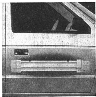
Carrosserie à structure renforcée, avec renforts contre les collisions latérales.
