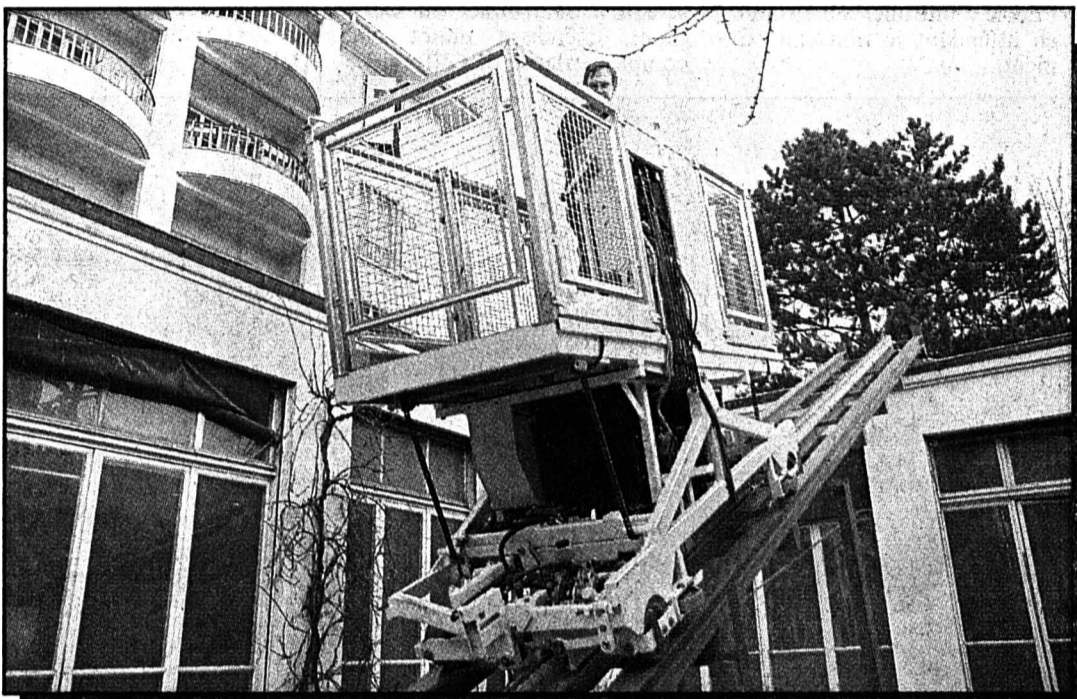
Un funiculaire pour permettre la maintenance des cheminées d'aération. (Comtesse)
