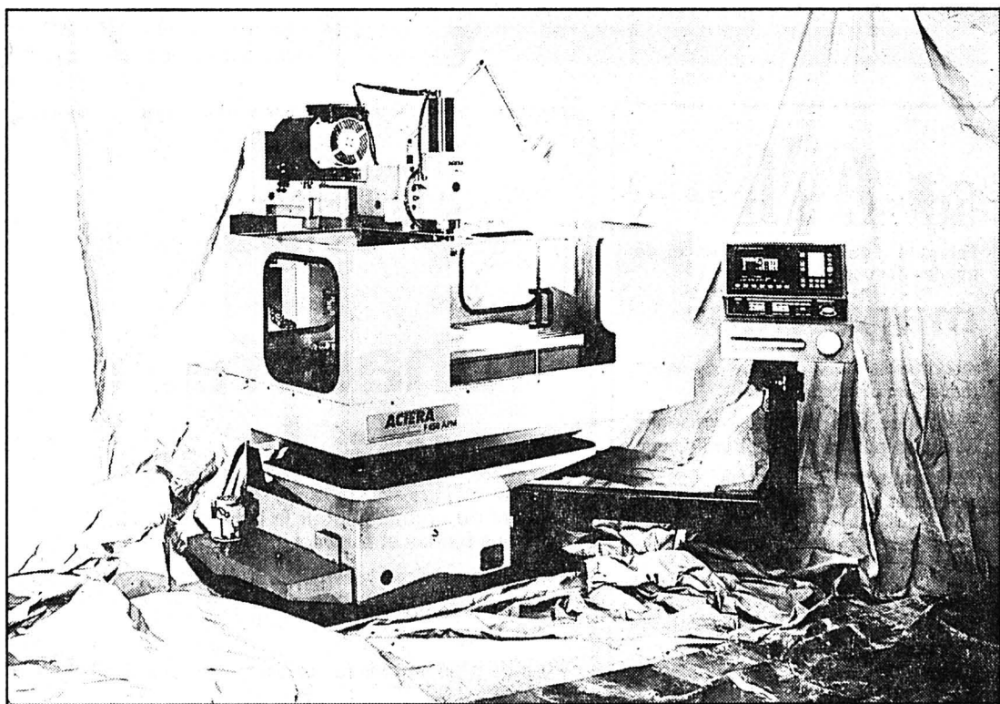
La F450 APM d'Aciera: une fraiseuse pour la mécanique générale de précision.
