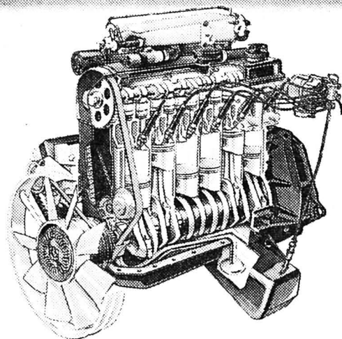
VW LT. 6 cylindres à injection d'essence.
