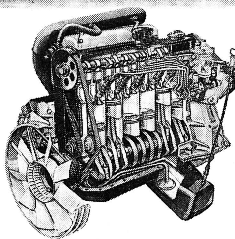
VW LT. 6 cylindres turbo diesel.
