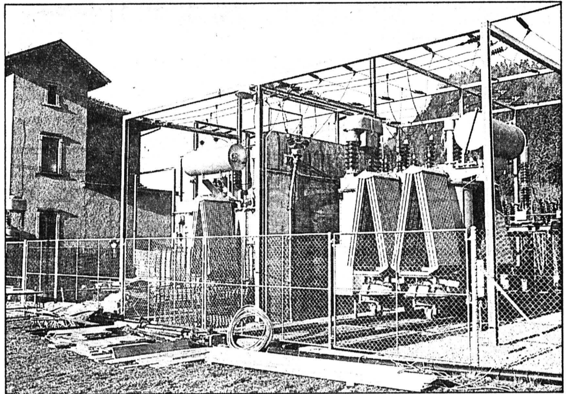
Les deux transformateurs à la station de Môtiers. C'est celui de droite qui a lâché... (Photo Impar-Charrère)
