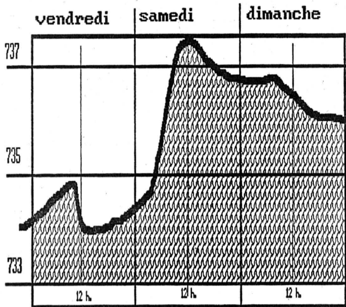
Niveau de la nappe dans le puits du pompage de Fleurier. Élévation de plus de deux mètres le 26 septembre 1987.
