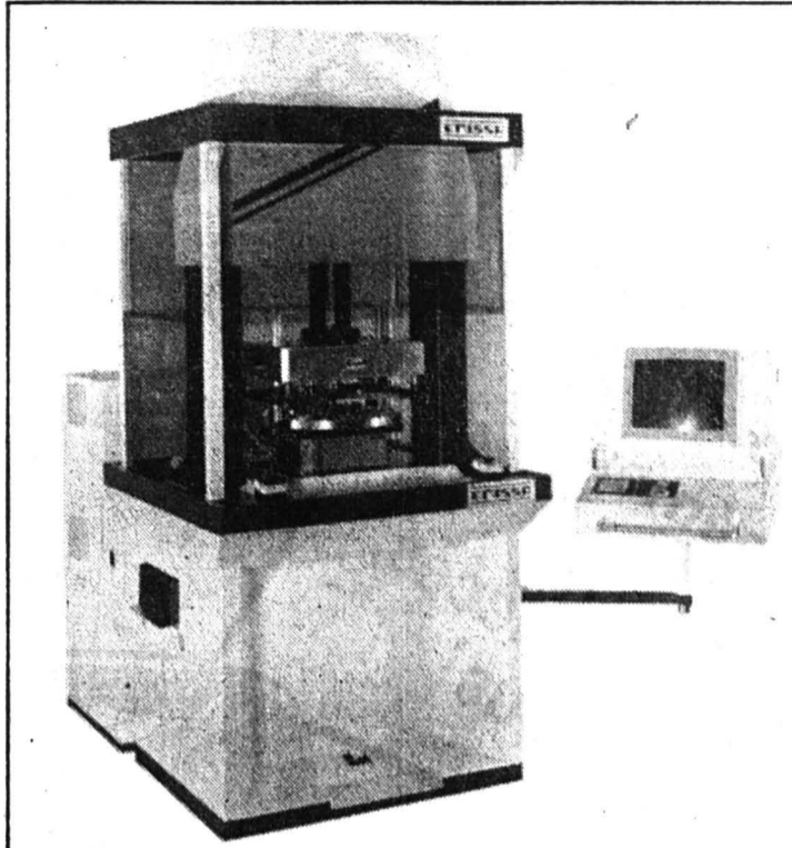
La MP 600 d'Emissa, la nouvelle ligne de machine flexible de production.
