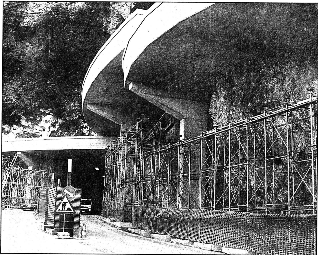
Les ouvrages de protection contre les chutes tels qu'ils ont été découverts ces derniers jours. (Photo Impar-Perrin)
