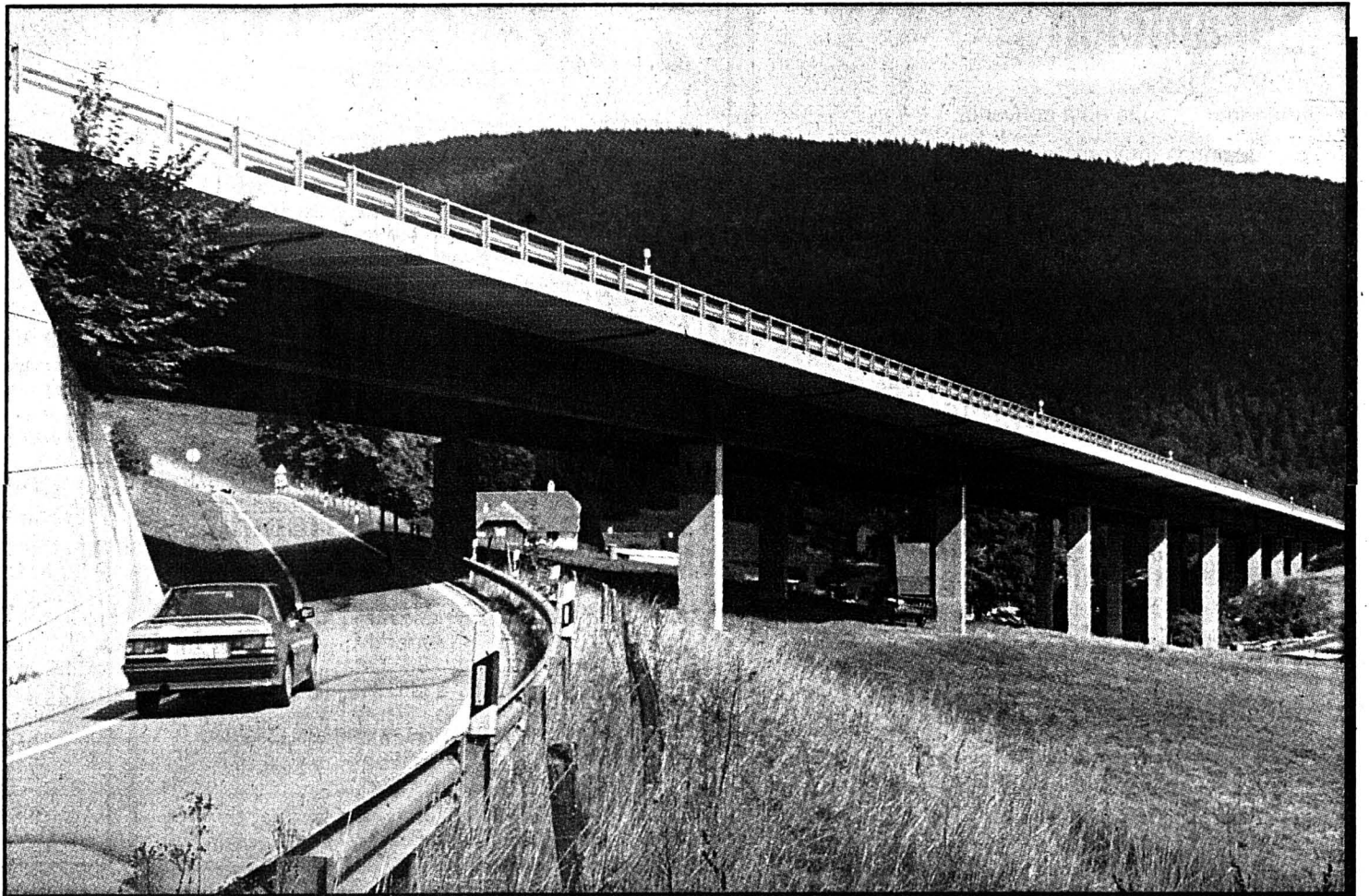
PBR Le viaduc de Valangin: un examen de routine pour pont de sinistre mémoire.
