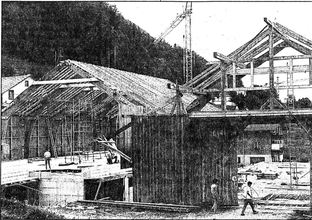
Effectué avec un camion-grue de 40 tonnes, le déménagement de la charpente, entre l'ancien bâtiment (à droite) et le nouveau, devrait être achevé aujourd'hui à midi.
