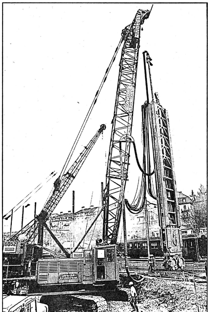
L'hydrofraise en action sur le chantier Migros: pour la première fois en Suisse. (Photo Impar-Gerber)
