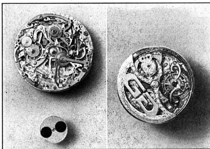
Montre poignet avec tourbillon de Gérald Genta. Un petit bijou!
