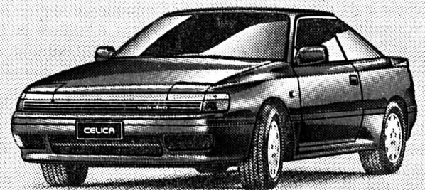
Celica Turbo 4WD: 3 portes, 4 places, 4 cylindres, 1998 cm 3 , 136 kW (185 ch) DIN, 16 soupapes, 5 vitesses, turbocompresseur à échangeur, transmission intégrale permanente, freinage antiblocage, fr. 41 200.-. Celica 2.0 GTi , fr. 28 900.-.
