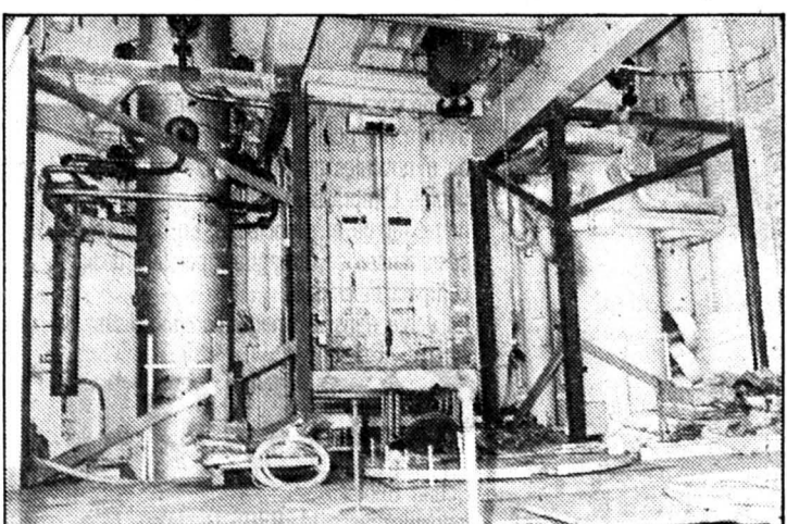
Le réacteur de la centrale expérimentale de Lucens. (Bélino AP)
