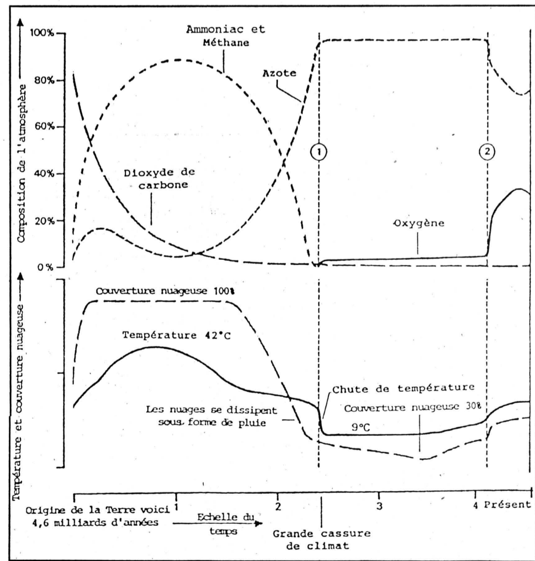
Fig. 2: Evolution aproximative de l'atmosphère terrestre, depuis la formation du globe à nos jours. Vers 2,4 milliards d'années, l'atmosphère est devenue oxydante et la végétation a pu sortir des mers. Mais c'est aux environs de 4 milliards d'années seulement que le taux d'oxygène a augmenté suffisamment pour permettre à un écran d'ozone de se former en altitude, capable de retenir les rayons ultra-violet. Dès ce moment, les animaux ont pu sortir des océans et prendre possession des terres émergées [graphique adapté de M. H. Hart, «The evolution of the atmosphere», Icarus vol. 37, p. 23 (1978)].
