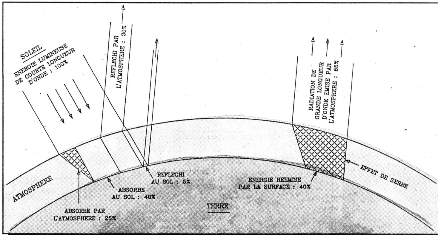
Fig. 1: Equilibre énergétique entre la radiation lumineuse reçue du Soleil, principalement aux longueurs d'ondes de la partie visible du spectre, et celle réémise par la Terre dans l'infrarouge. 35% environ de l'énergie solaire incidente sont renvoyés directement vers l'espace, comme par un miroir. Ce rapport constitue ce qu'on entend par albédo moyen de la planète Terre.
