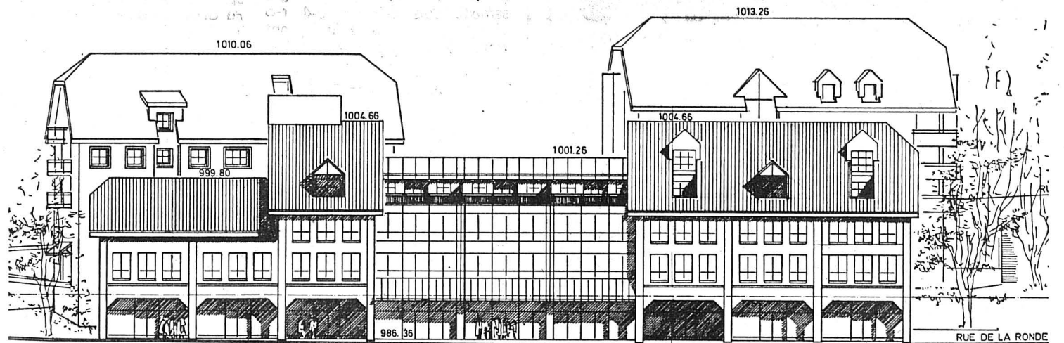
La façade nord du complexe projeté avec sa galerie commerciale au rez, sur la rue de la Ronde.
